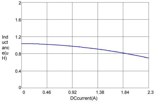
SMDH3010TF-1R0
