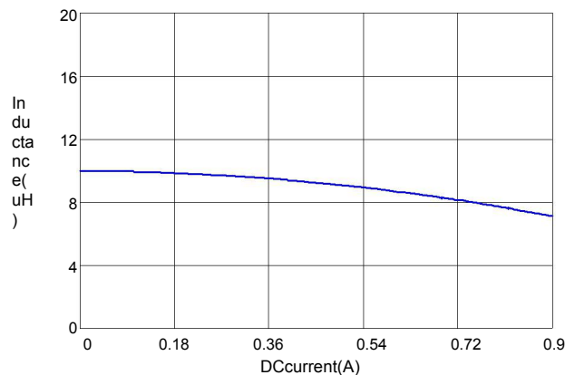
SMDH3010TF-100
