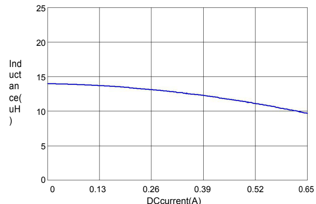
SMDH3010TF-150
